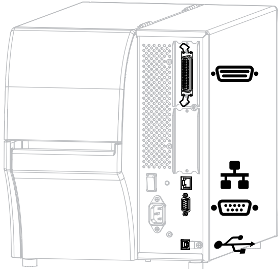
그림 14 통신 인터페이스의 위치
