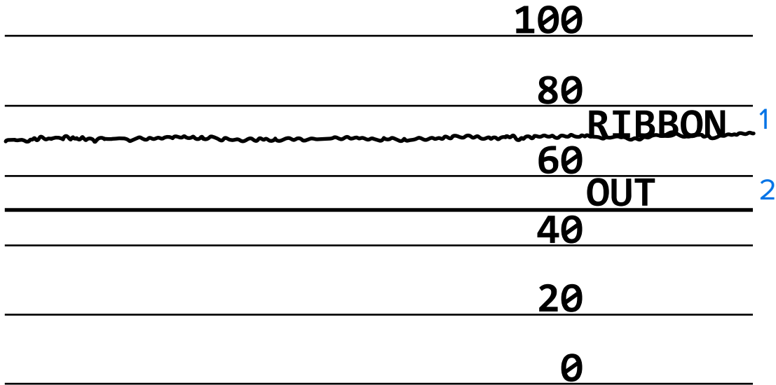
그림 7 센서 프로파일(리본 섹션)
