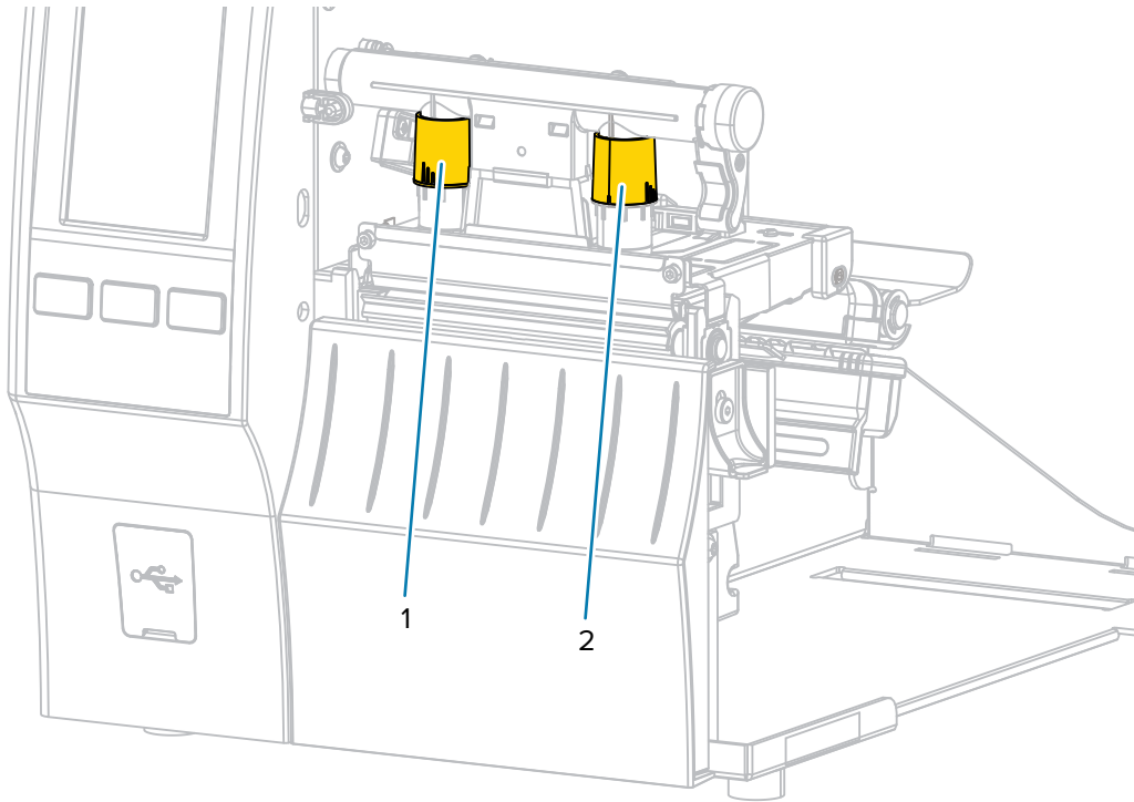
그림 2 인쇄헤드 압력 조정 다이얼
