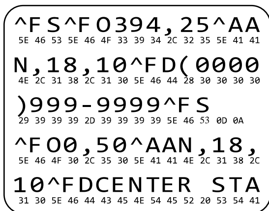
图 11 通信诊断模式标签样例
