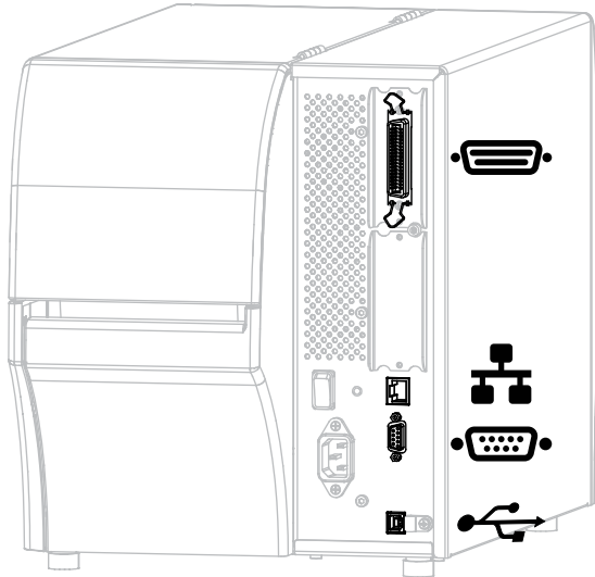
图 15 通信接口位置
