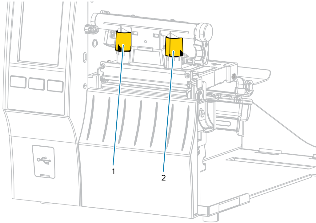
그림 3 인쇄헤드 압력 조정 다이얼
