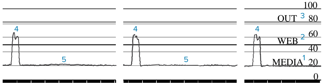
그림 10 미디어 센서 프로파일(블랙 마크 미디어)
