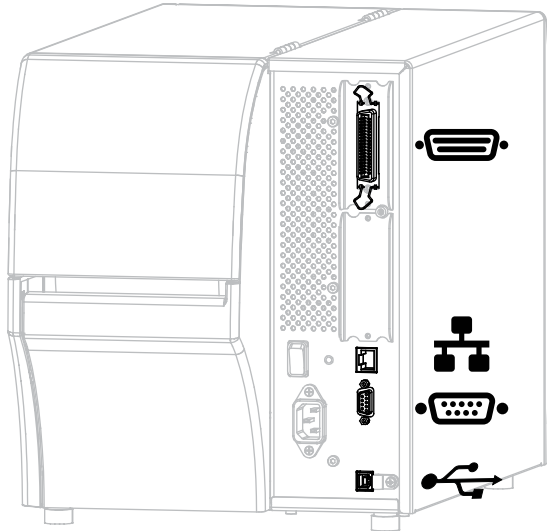
그림 15 통신 인터페이스 위치
